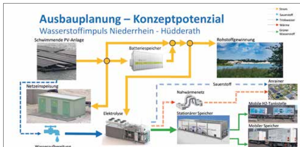
Der überschüssige Energieanteil wird mittels Elektrolyse in grünen Wasserstoff umgewandelt und gespeichert. Der Energieträger steht weiteren Unternehmen zur Verfügung.
