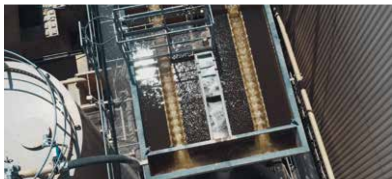
Das Tunnelmaterial durfte nicht im offenen Waschwasserkreislauf gereinigt und klassiert werden. Das vorhandene Kieswerk musste um einen geschlossenen Waschwasserkreislauf erweitert werden.
